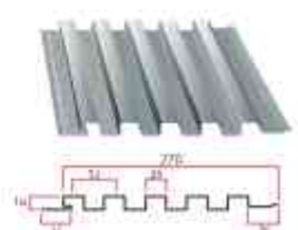
ลอนNova-Panel III
