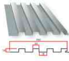
ลอนNova-Panel II
