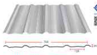
ลอนT-ONE 760B (กลิ้งฝ้า)
