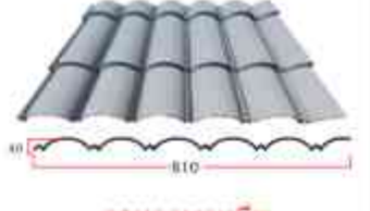
ลอนวาเลนชัย
