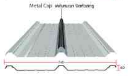
ลอนNova Lock Vit 740
