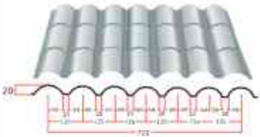
ลอนนิบูน
