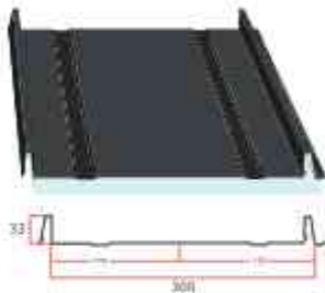
ลอนNova-Cooling Snap
