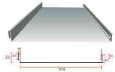
ลอนNova-Major Snap
