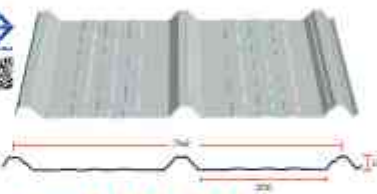
ลอนT-ONE 760C (3 สันลอน)
