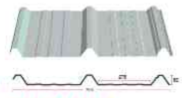
ลอนT-ONE 740-50 (3 สันลอนสูง)
