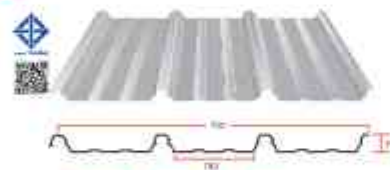
ลอนT-ONE KL700 (kloplok)
