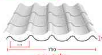
ลอนแสง
